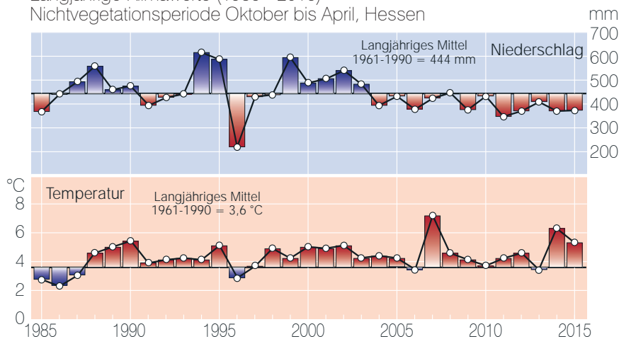
Langjährige Klimawerte (1985 - 2015)
