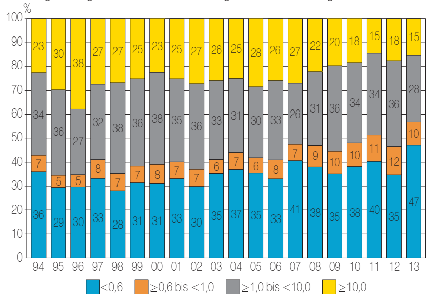
Tiefenunabhängiges Bc/Al-Verhältnis in der Bodenlösung. Datengrundlage: 37 Intensiv-Monitoringflächen, Zeitbezug: 1994-2013
