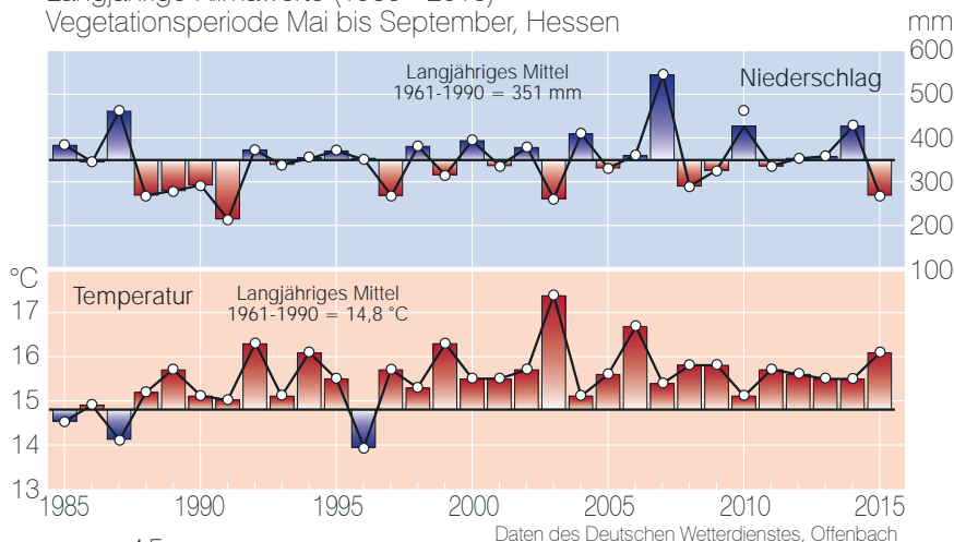
Langjährige Klimawerte (1985 - 2015)
